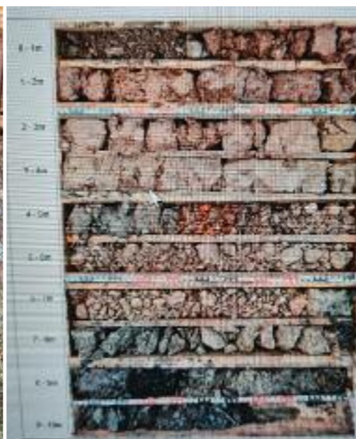
Brunnenöffnung zwischen Platz 4 u. 5 Schichtmaterialien für die geologische Untersuchung
